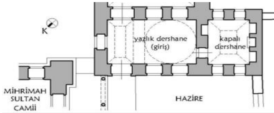
(شكل ٢٨) مسقط أفقي لمكتب صبيان مهرمه سلطان بإدارة قاضي - نقلاً عن :
