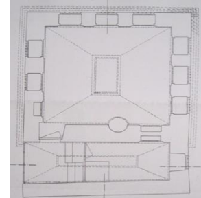
(شكل ٢٢) مسقط أفقي لمكتب صبيان
