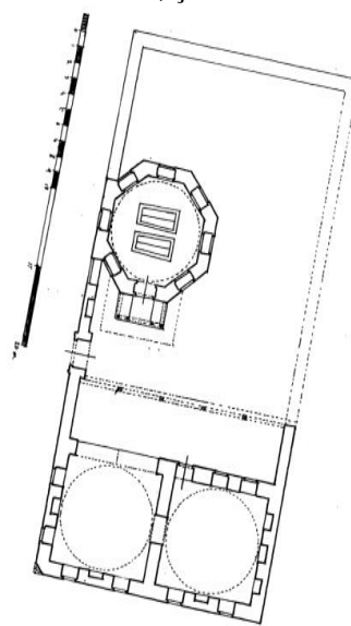
(شكل ٧) مسقط أفقي لكتبة شاه خاتون وما بها من مكتب - نقلاً عن : ÖZTURNA, F, «Sinan Dönemi Sıbyan Mektepleri», Sanat Tarihi Yüksek Lisans Tezi, Sosyal Bilimler Enstitüsü, İstanbul, 1991.
