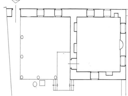
(شكل ٢٥) مسقط أفقي لمكتب صبيان
