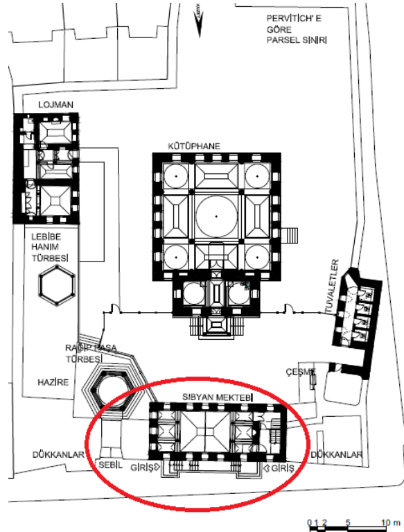
(شكل ١٦) مسقط أفقي لكلية قوجه راغب باشا وما بها من مكتب صبيان - نقلًا عن :
