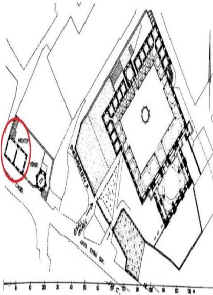
(شكل ٨) مسقط أفقي لكتبة قرا أحمد باشا وما بها من مكتب صبيان - نقلاً عن : FREELY, A History of Ottoman Architecture, 284, f.13.
