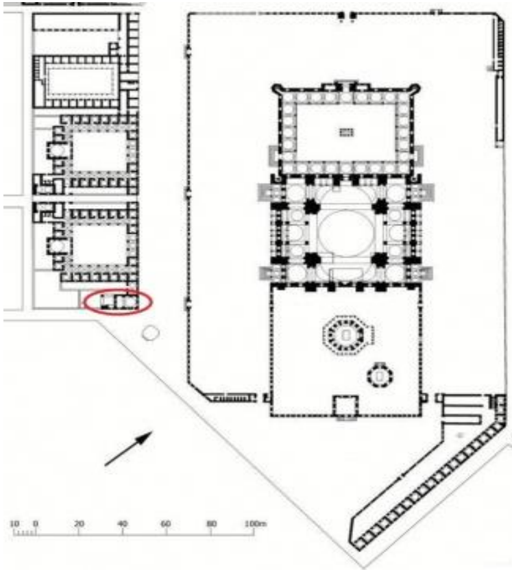
(شكل ١٢) مسقط أفقي لكلية السليمانية وما بها من مكتب صبيان - نقلاً عن :
