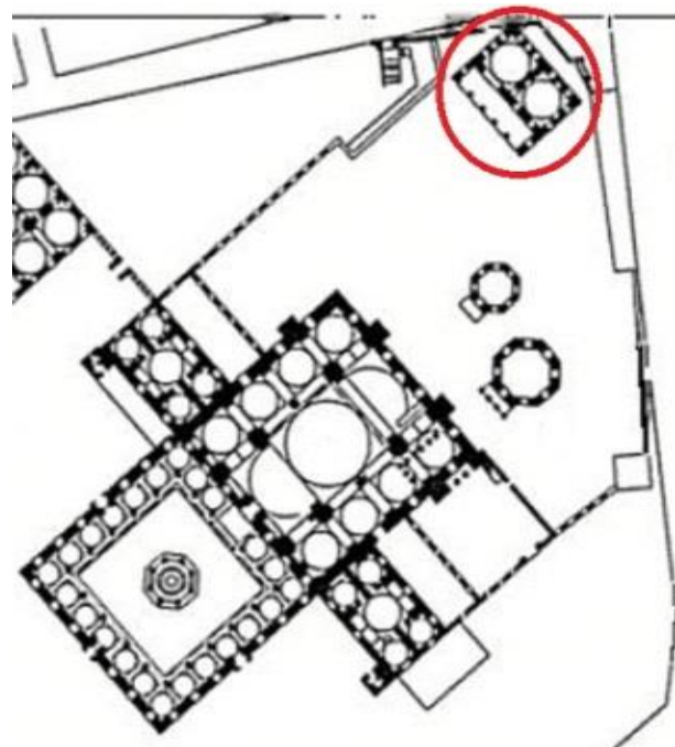
(شكل ١) مسقط أفقي لكلية بايزيد الثاني وما بها من مكتب
