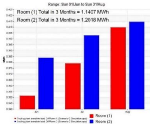
شكل (26): نتائج السيناريو الثاني: تحسين الأداء الحراري للنوافذ في الواجهة الجنوبية والغربية باستخدام الزجاج مزدوج المعالج بتقنية النانو (U-Value 1.5330 W/m2.K)
