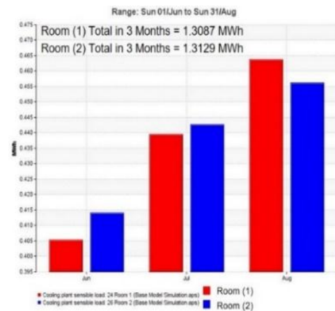
شكل (24): نتائج الحالة الأساسية (Base Model) لحساب حمل التبريد خلال الفترة الحارة (يونيو- يوليو- أغسطس) للغرفتين (1) و (2) (U-Value 5.7780 W/m2.K)
