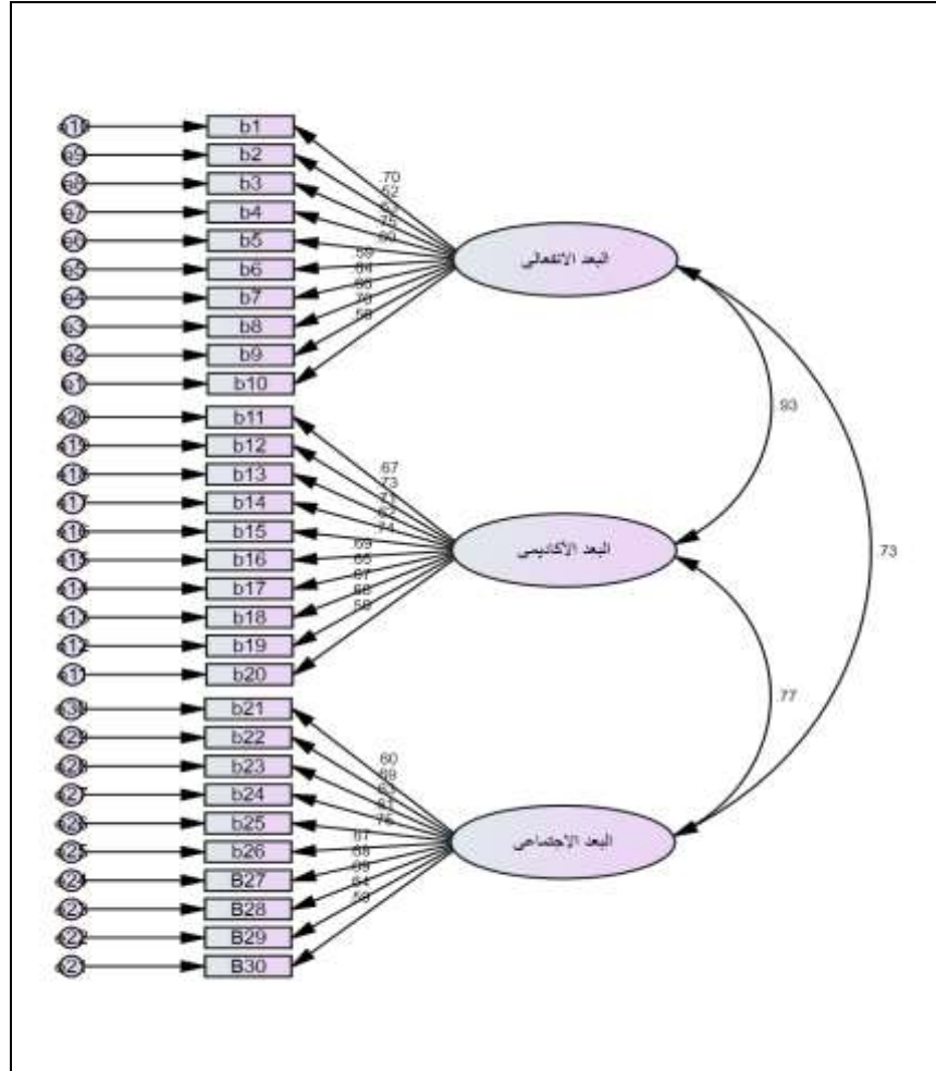
شكل ( ٢ ) البناء العامي لمقياس التوافق النفسي
