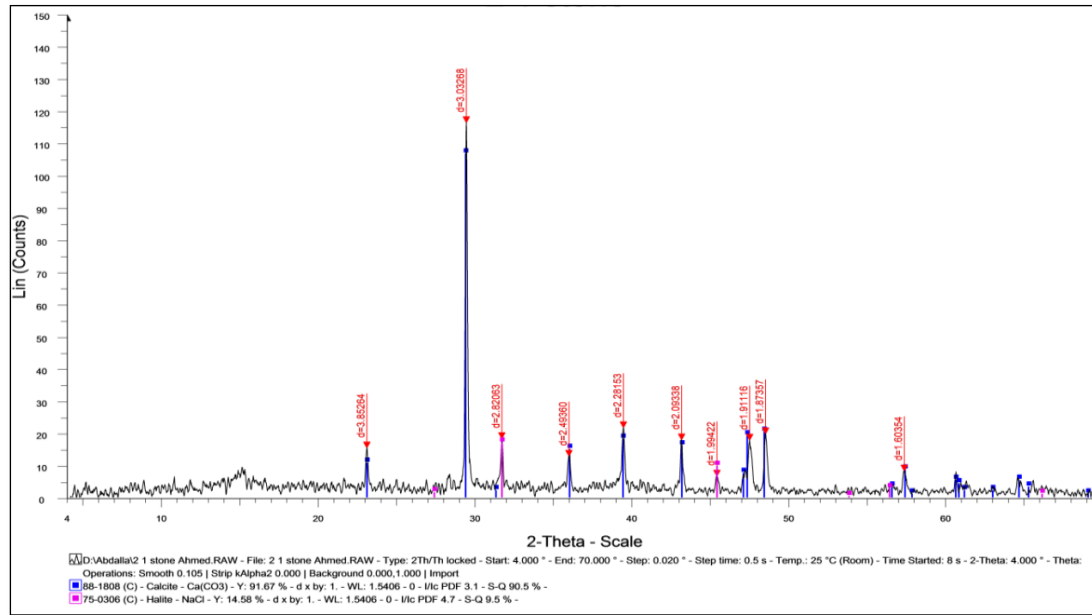
(شكل ١) يمثل نمط حيود الأشعة السينية (XRD) لعينة من الحجر الجيري بمعبد حريشاف © عمل الباحث
